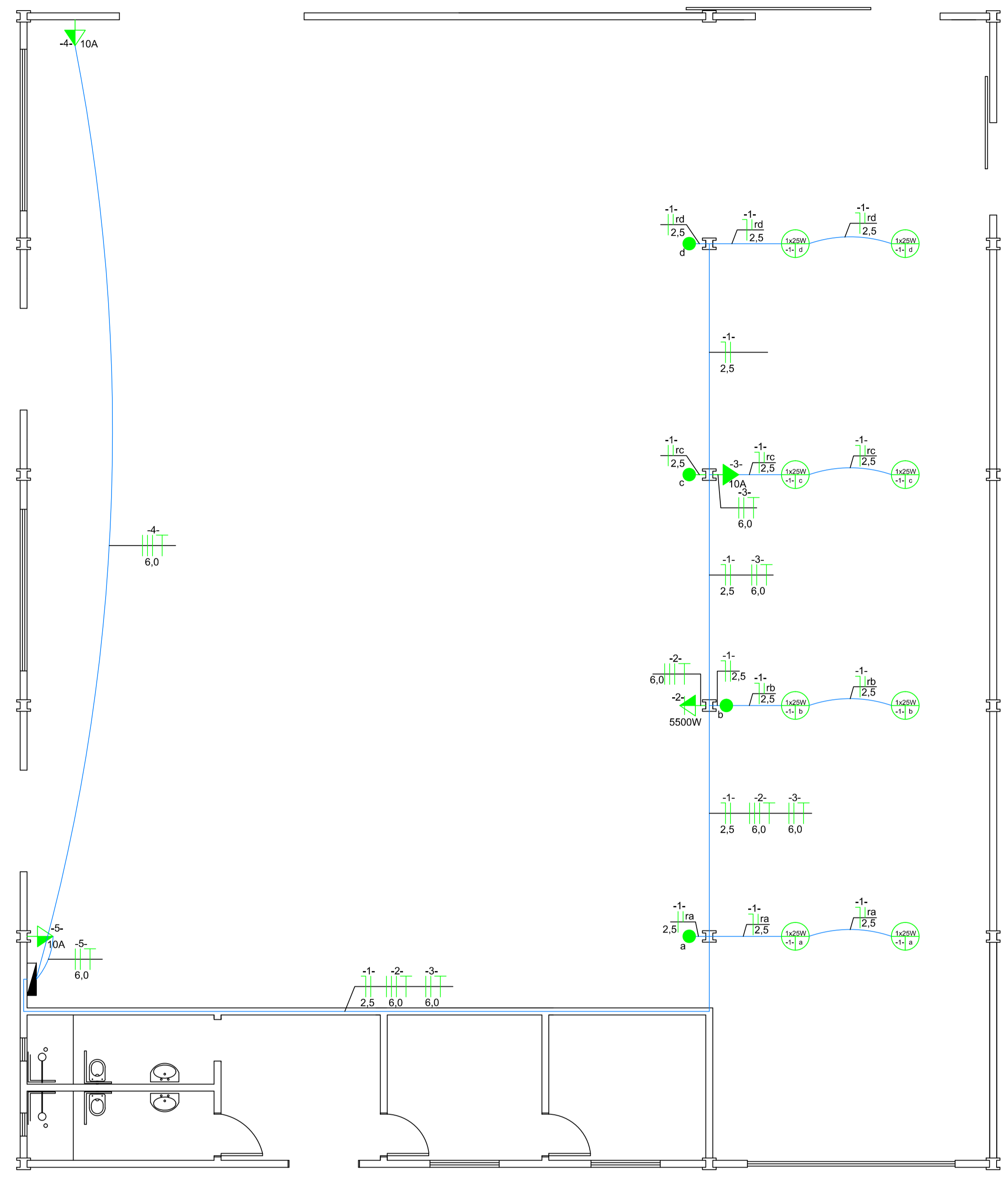
PLANTA BAIXA ELÉTRICO ESC. 1/75
